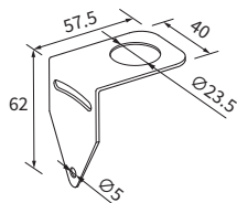
O30 brackets
